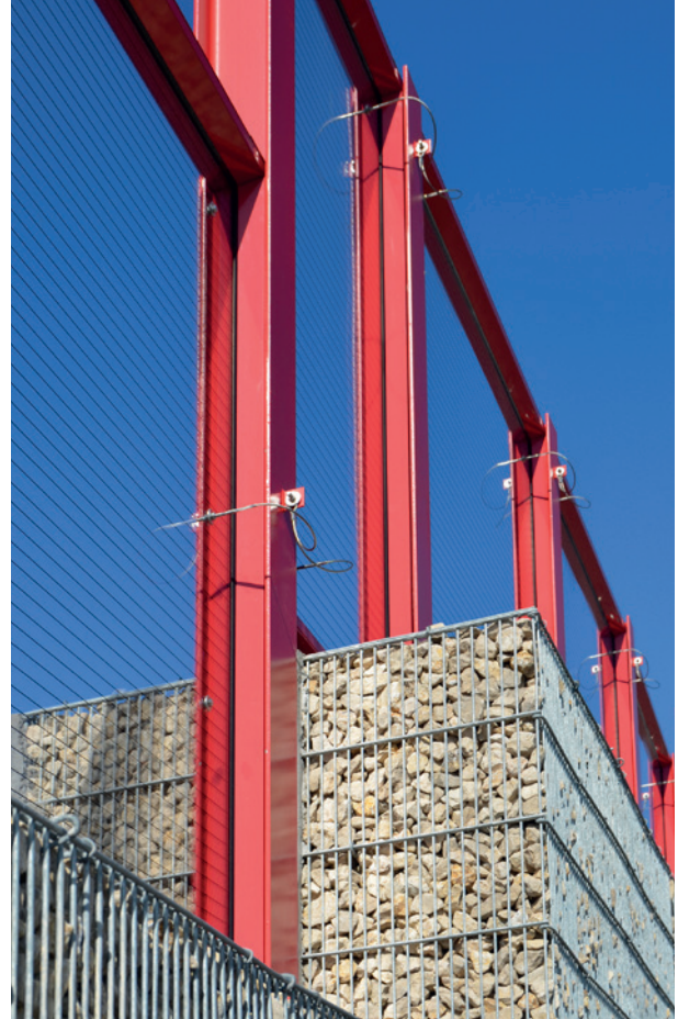
Lärmschutzwand, Pirmasens PLEXIGLAS® Soundstop GS CC, 15 mm
