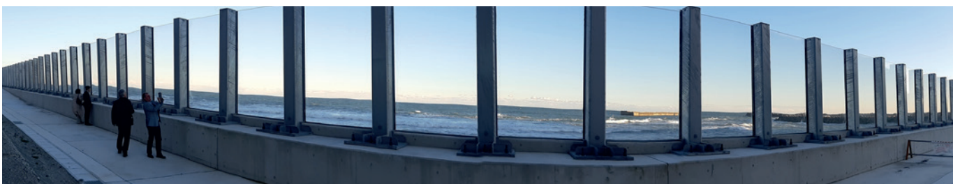
Lärmschutzwand, Fukushima Tsunami barrier
