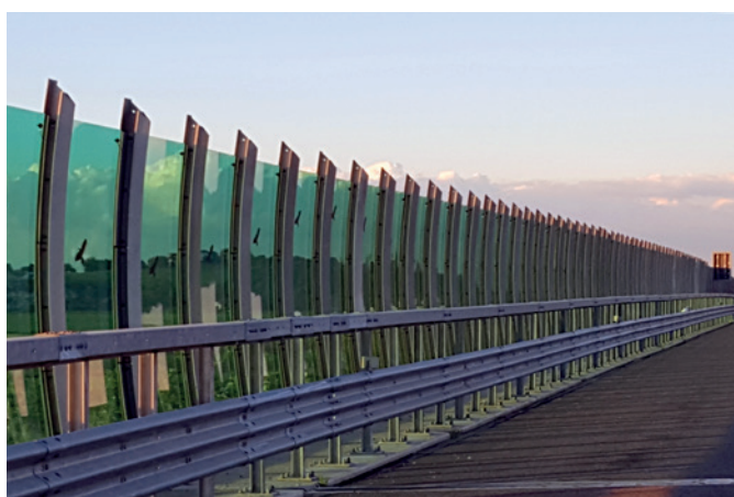
Lärmschutzwand, Autobahn Valdastico Sud PLEXIGLAS® Soundstop XT 20 mm, Spring Green Valdastico
