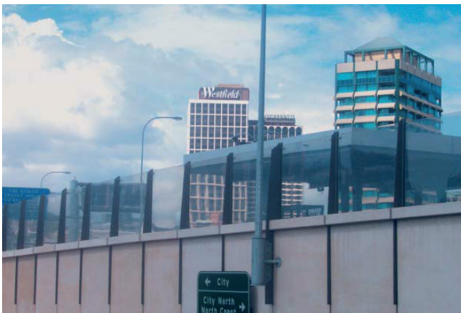
Lärmschutzwand, Eastern Distributor, Sydney PLEXIGLAS® Soundstop XT und GS CC Leighton Constructions
